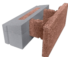
Steigungsblock
